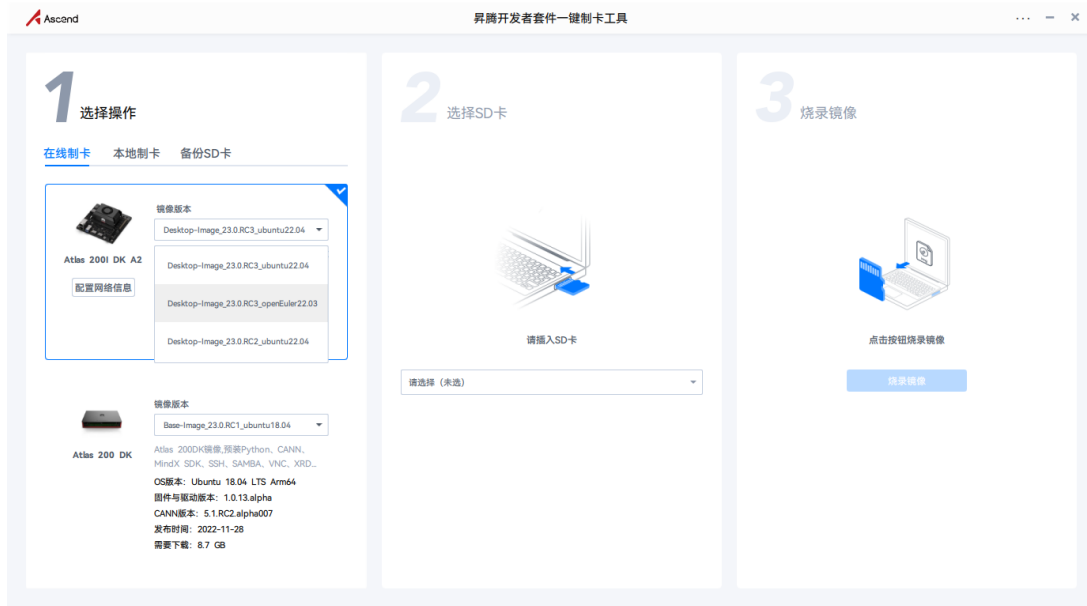
图 3-3 一键制卡工具界面图
