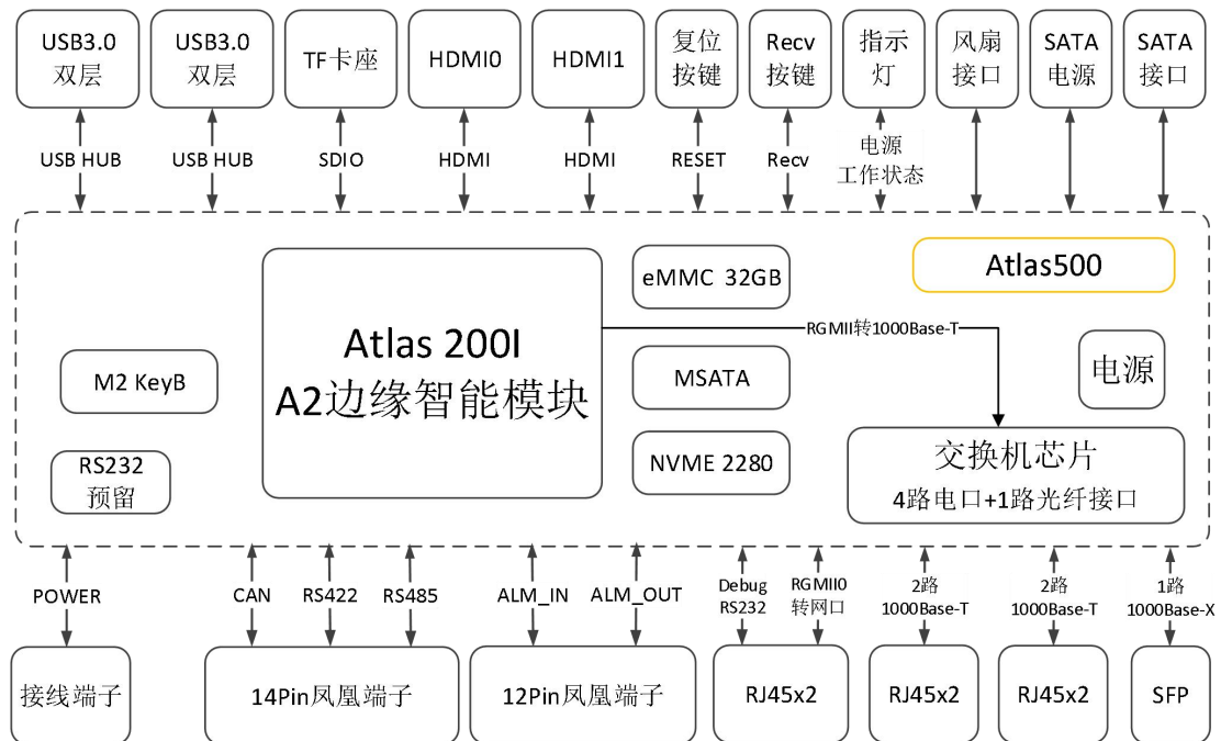
图 1-6 QA500A2-B 系统框图
