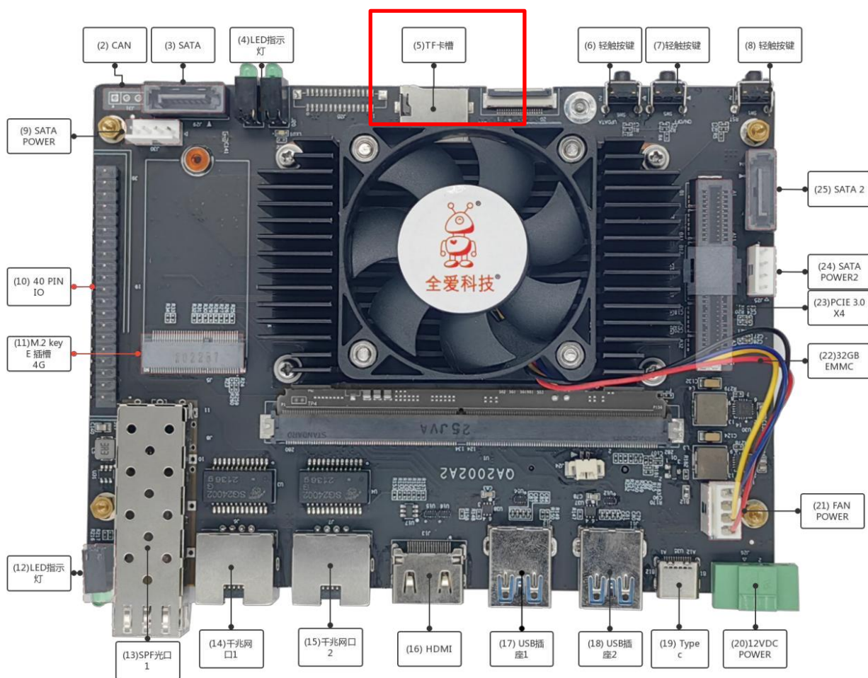
图 4-1 插入 SD 卡
