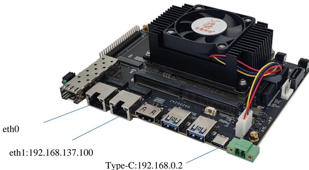
图 3-6 开发者套件各接口默认 IP 地址
