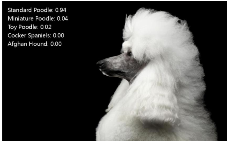
图 8-2 推理结果
