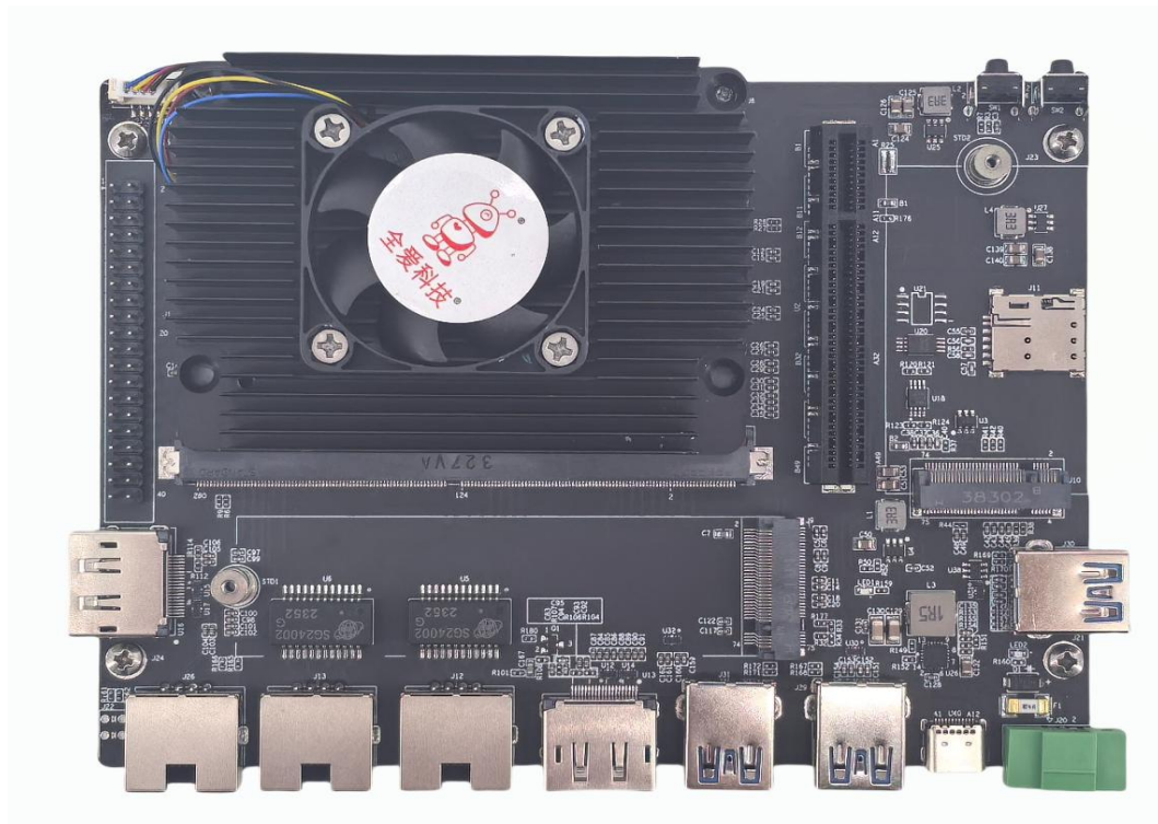
图 1.1 外观图
