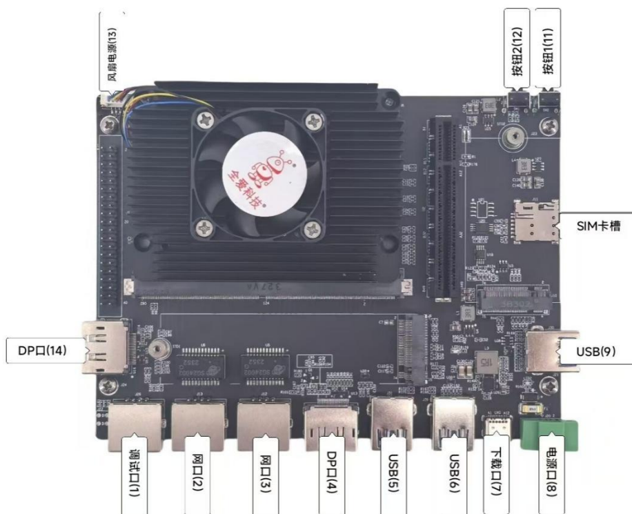
图 1.2 正面引脚图
