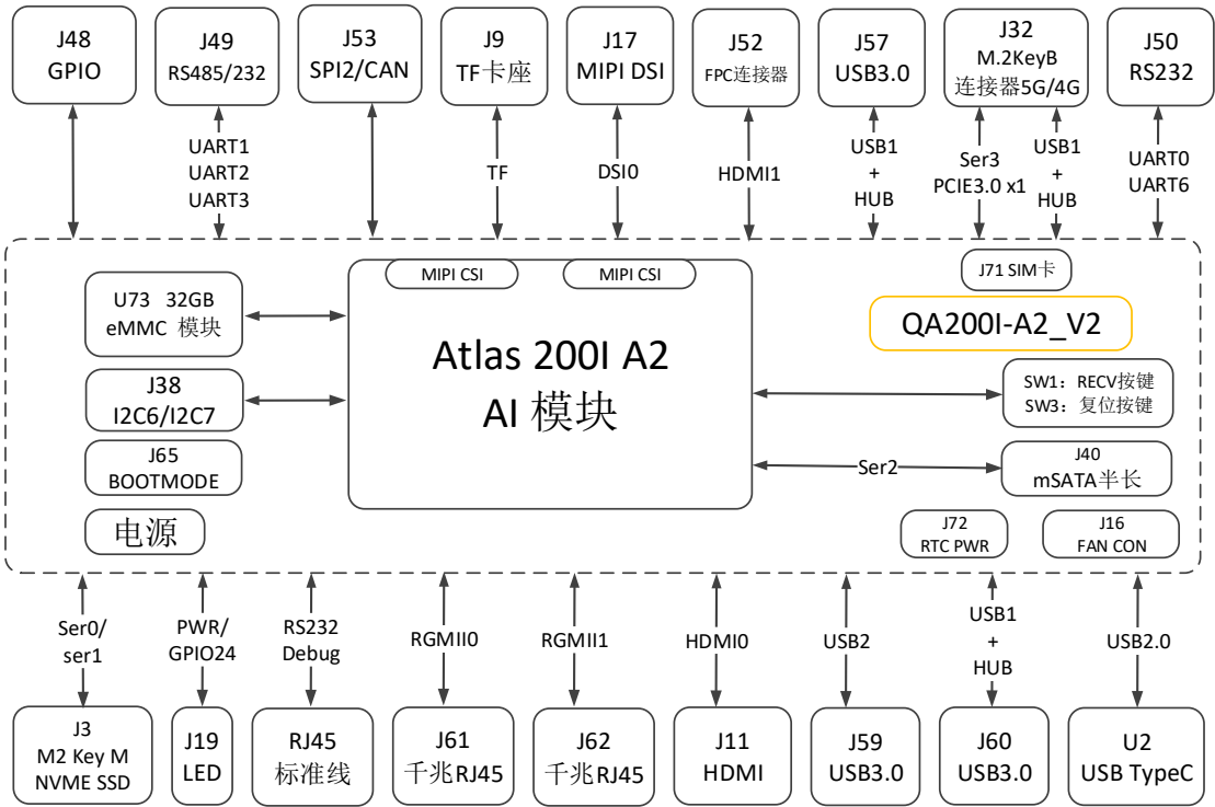
图 1-4 后羿智盒系统框图
