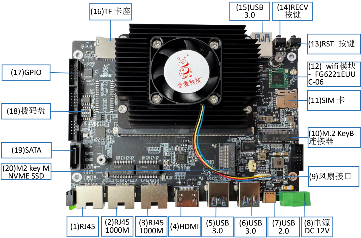
图 1-3 按键与接口说明
